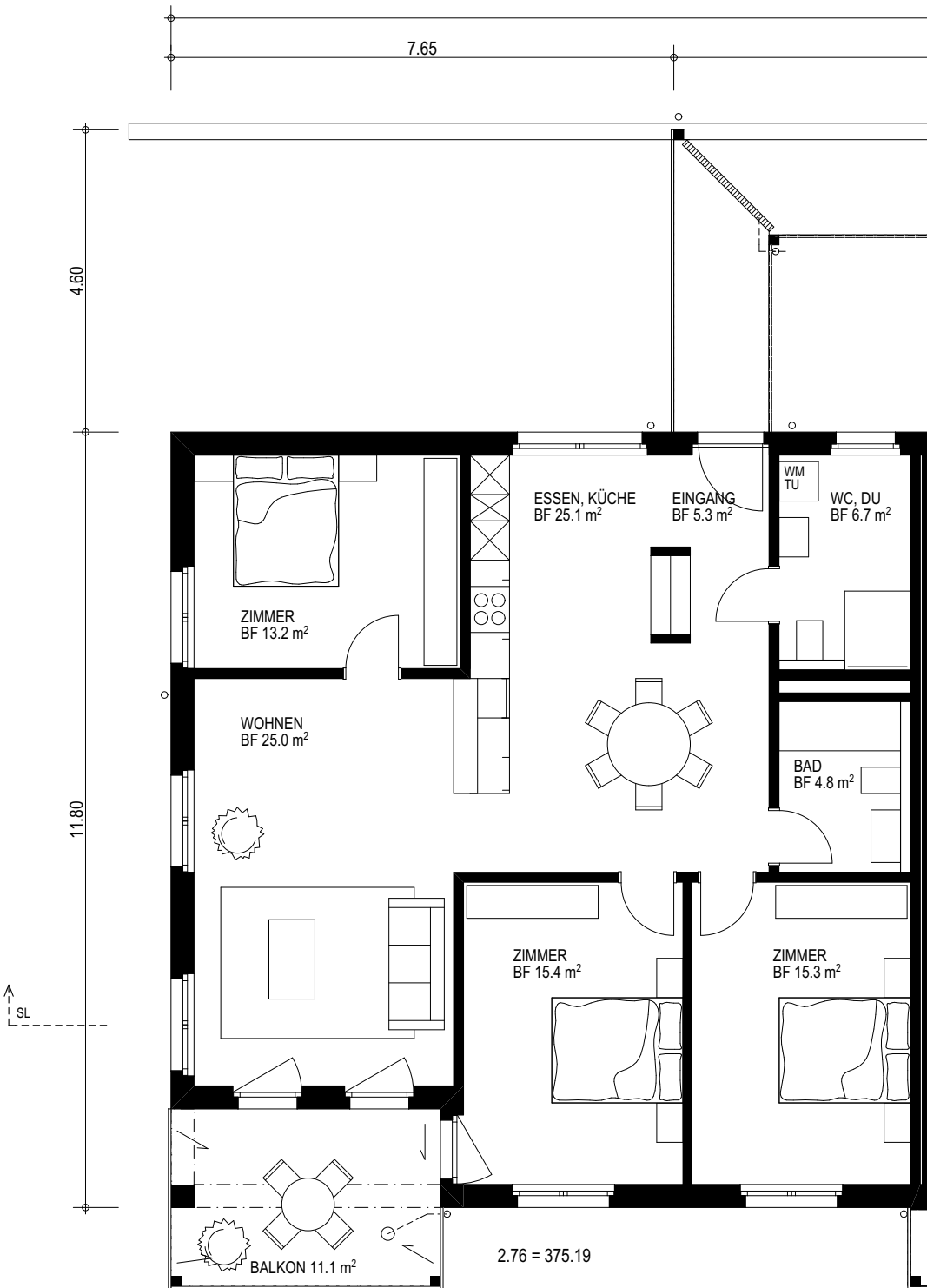
W04 4/5 ZI 115.0 m 2 AUSSENFLÄCHE 11.1 m 2
